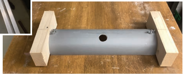
In de pvc pijp een gat geboord en daarna in de lengte door midden gezaagd en d.m.v. een slotboutje en vleugelmoer de pijp op de halve cirkels gemonteerd. Let op De buis moet langer zijn dan de breedte van de schuurplank.
